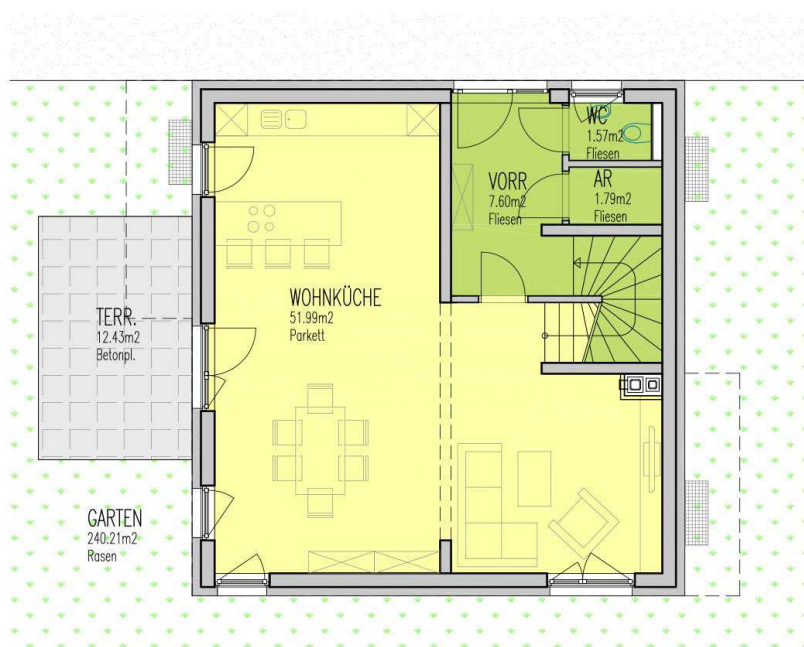
ERDGESCHOSS
