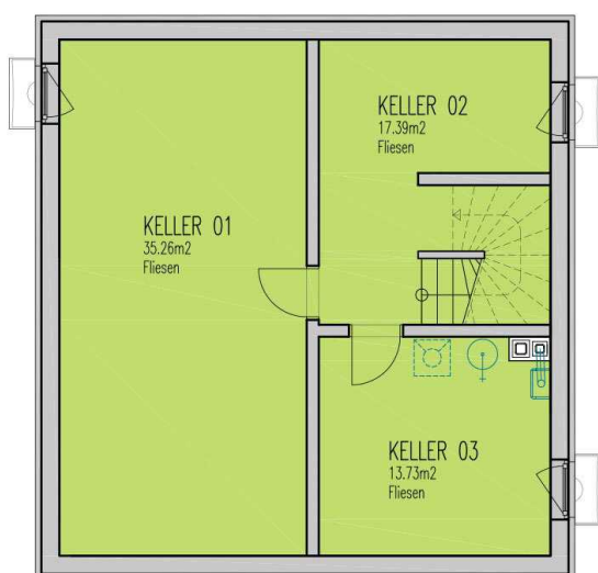
KELLERGESCHOSS
