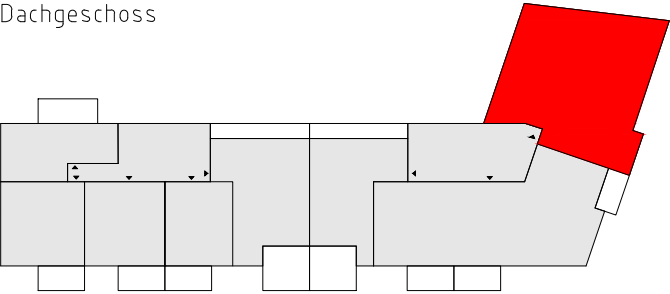
Dachgeschoss
