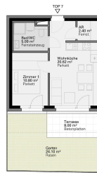
ERDGESCHOSS, STG 1, TOP 7
